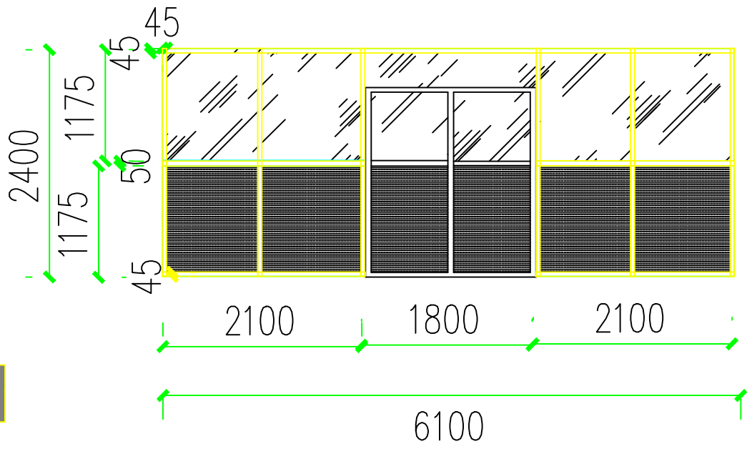
隔断立面图
